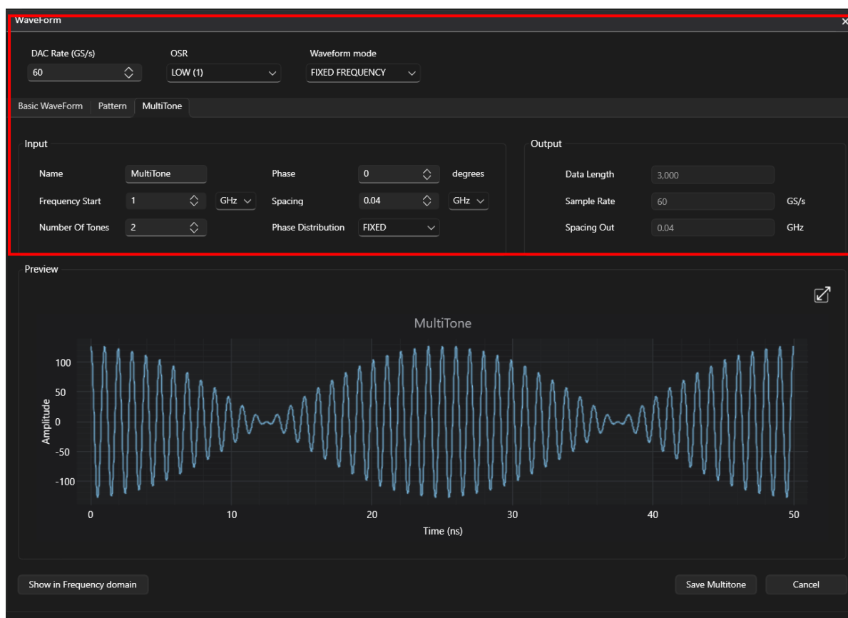
Figure 34: Multitone parameters
